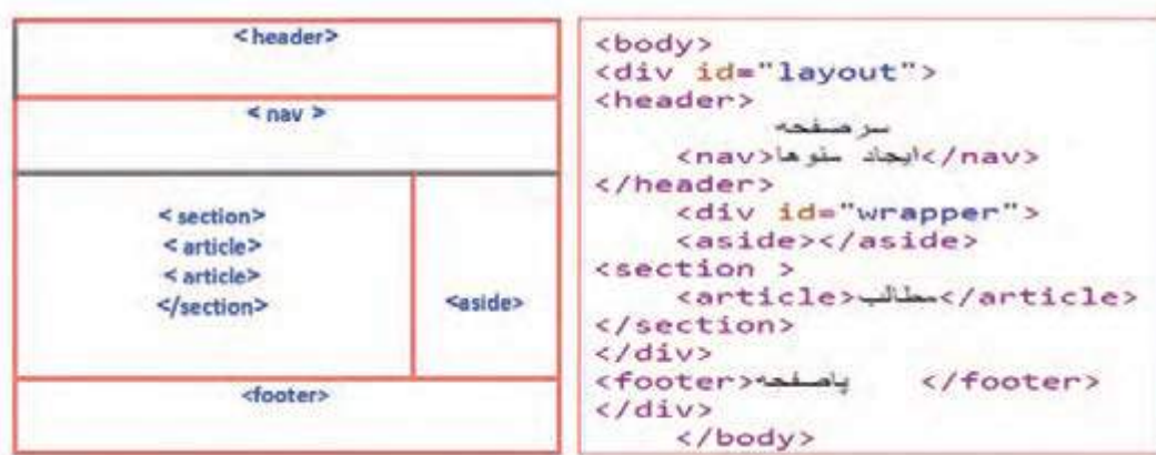
شکل ۱۶- ساختار html5
