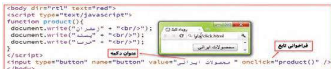
شکل ۶- رویداد onclick
