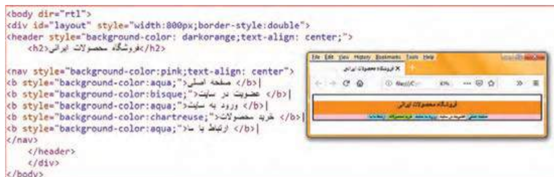
شکل ۱۸- پیام خطا
