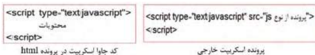
شکل ۳- ساختار script
