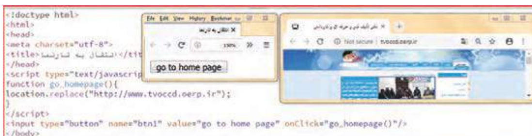
شکل ۸- متد replace
