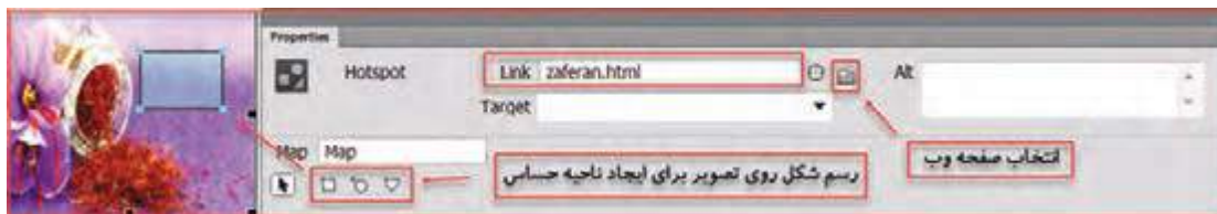
شکل ۴۳- ایجاد hotspot
