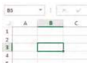
شکل ۲- سلول فعال
